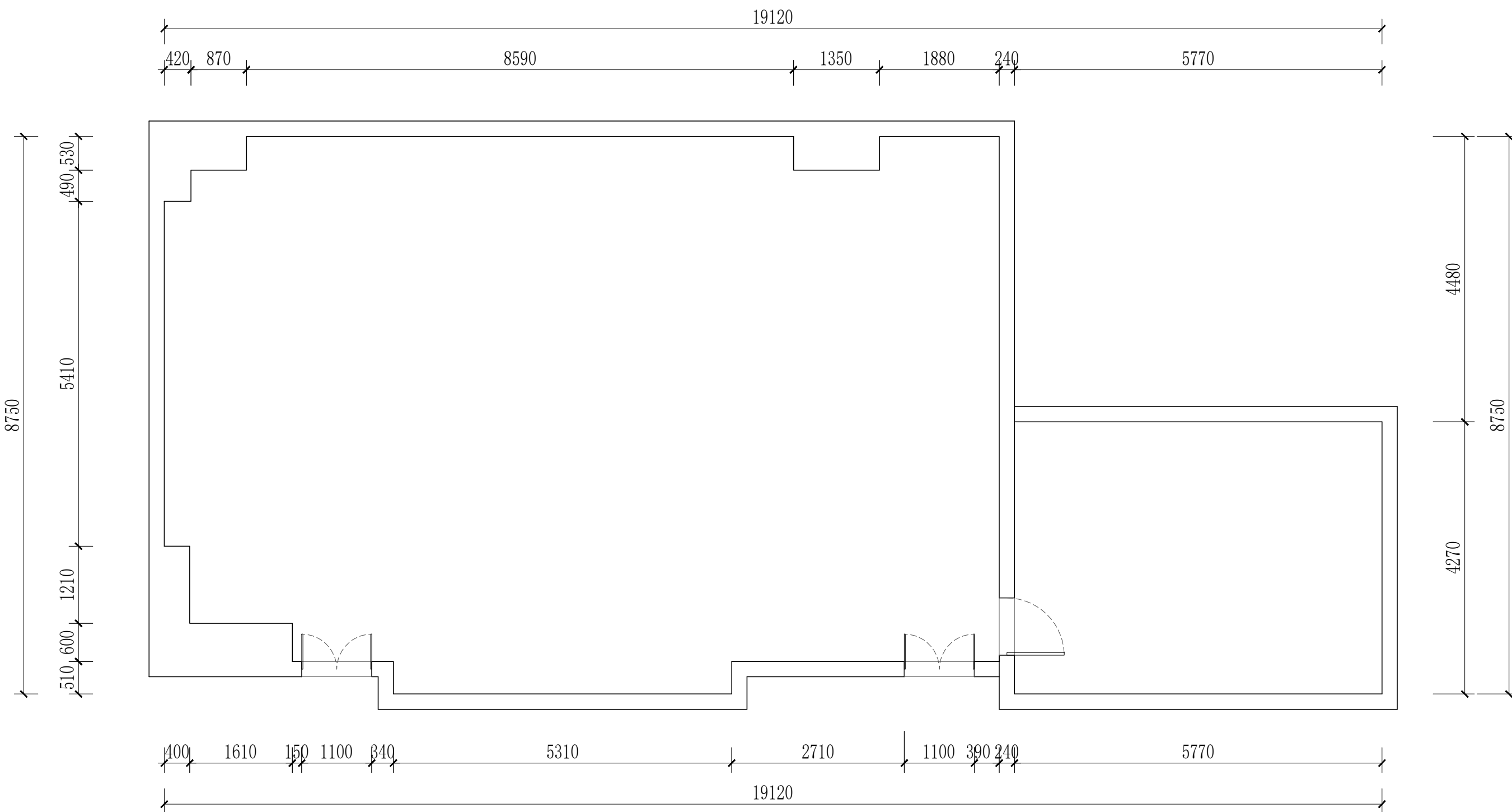
B 4 0 3 \ B 5 0 3 办公室尺寸图
